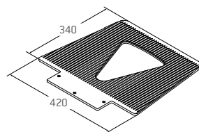
Bavette G (420x340x7 mm) pour les palettes grand format Réf. 930 003
