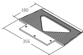
Bavette WL (356x180x7 mm) notamment pour le gros électroménager et le remplissage des machines automatiques, Réf. 930 018
