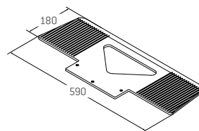
Bavette XWL (590x180x7 mm) convient également pour le gros électroménager, les pieds sont sur la bavette, Réf. 930 074
