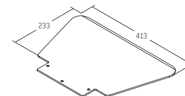
Bavette V (413x233x5 mm) pour le transport des bombonnes d'oxygène Réf. 930 001
