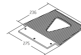
Bavette standard (275x236x7 mm) à rainures longitudinales, pour éviter un glissement latéral, Réf. 030 025
