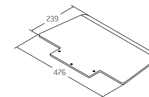
Bavette GS-NG (476x239x7 mm) pour les cartons (par ex.: cannettes) Réf. 930 084
