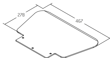
Bavette LH (467x278x5 mm) comme Bavette V, mais de plus grande taille Réf. 930 002
