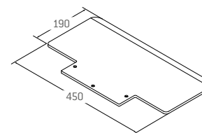
Bavette DS-NG (450x190x7 mm) ainsi que pour la centrale pour les cartons Réf. 930 085
